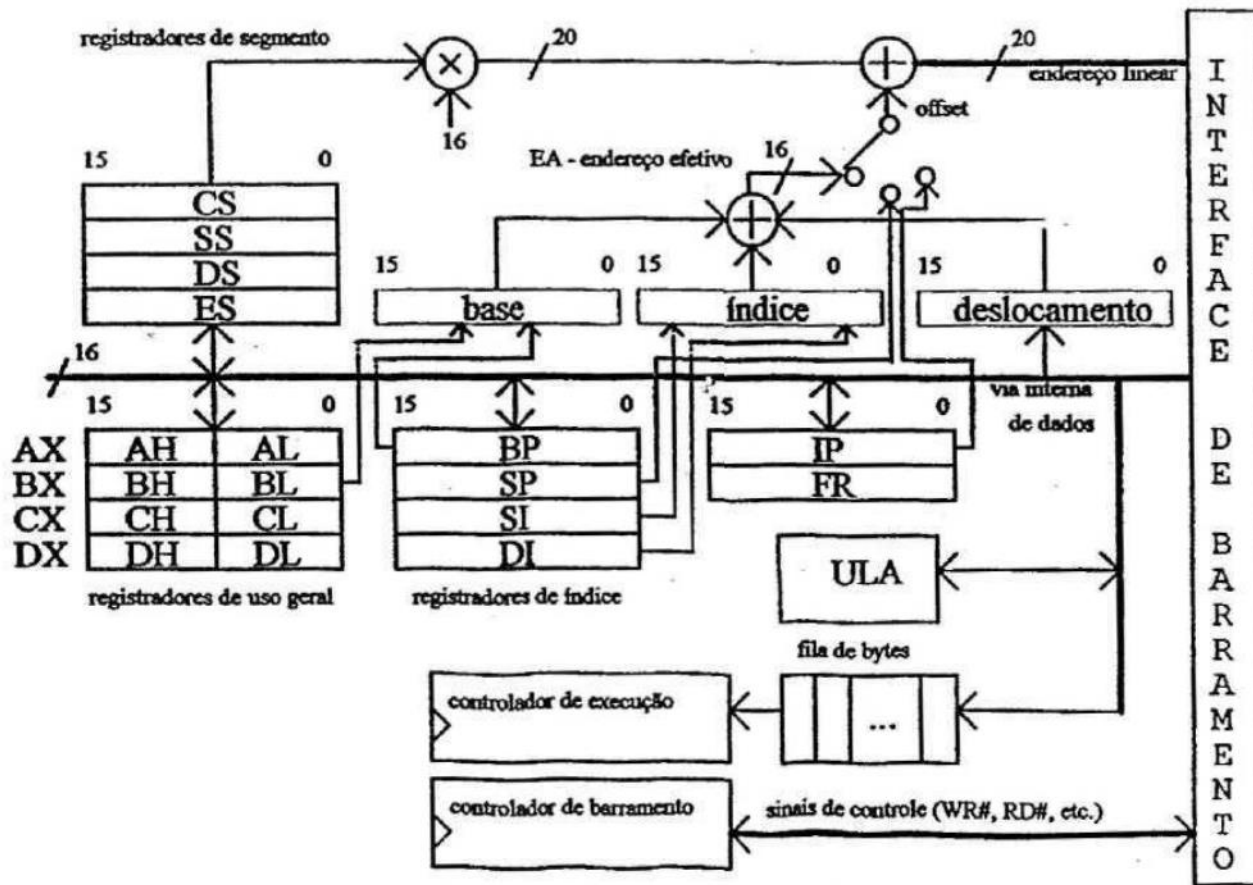
Figura 2.1 - Arquitetura interna simplificada do 8086/88.
